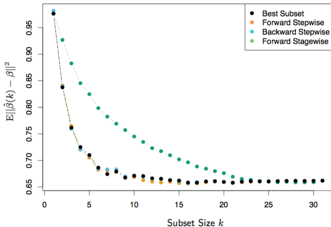
FIGURE 12 – Comparatives de méthodes stepwise . Comparaison de quatre techniques de sous-sélection des régresseurs soumis à un problème de régression linéaire : Y = X\beta + \epsilon . Il y a n = 300 individus avec p = 31 variables explicatives gaussiennes. Pour 10 variables, les coefficients sont tirés au sort à partir d’une loi \mathcal{N}(0, 0.4) , le reste est nul. Le bruit suit une loi normale \epsilon \sim \mathcal{N}(0, 6.25) . Les résultats sont moyennés sur 50 simulations. La figure montre l’erreur quadratique moyenne du coefficient estimé \hat{\beta}(k) à chaque étape contre la vraie valeur \beta [2].
