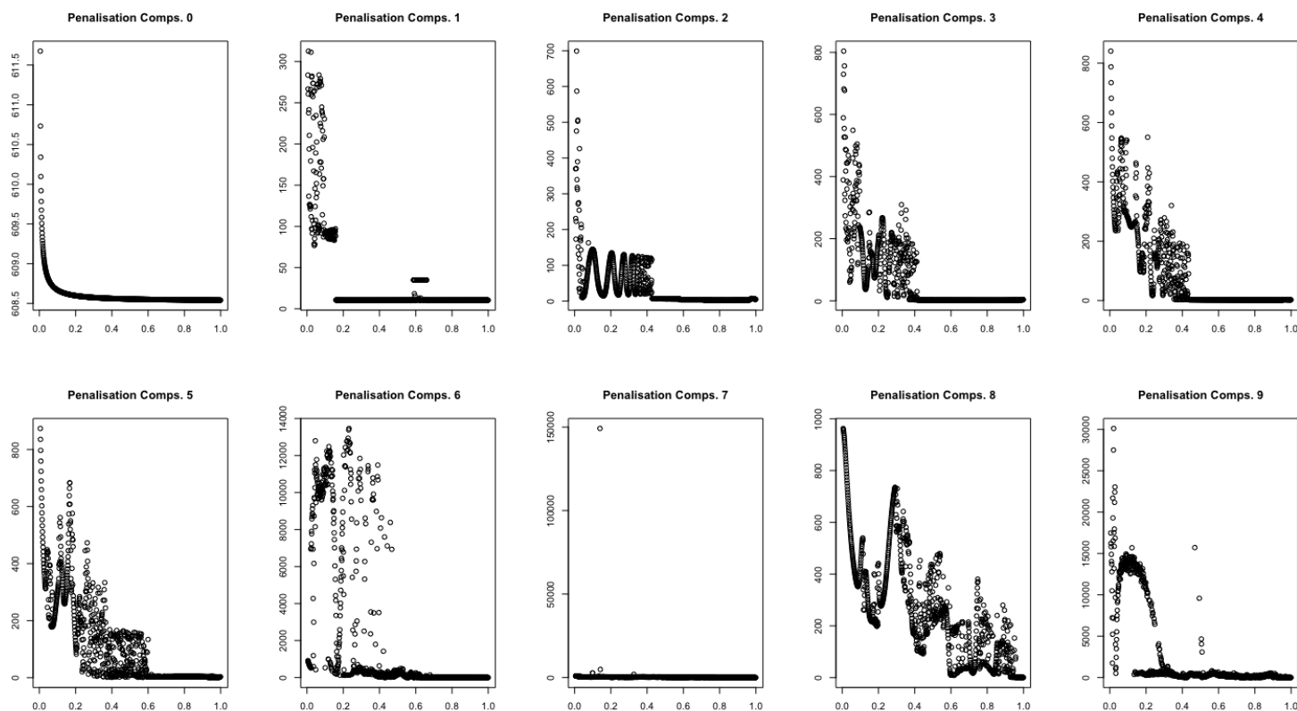
FIGURE 33 – Relation entre le paramètre de réglage de chaque régression et EMQ. Les abscisses dans la figure sont l'intervalle du paramètre de réglage, et l'ordonnées sont les erreurs quadratiques trouvées avec l'échantillon d'apprentissage.
